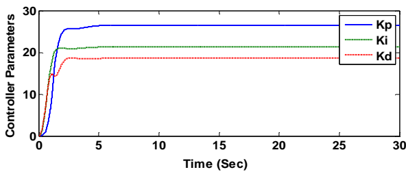
Fig. 8. The controller parameters trajectories using BSA.
